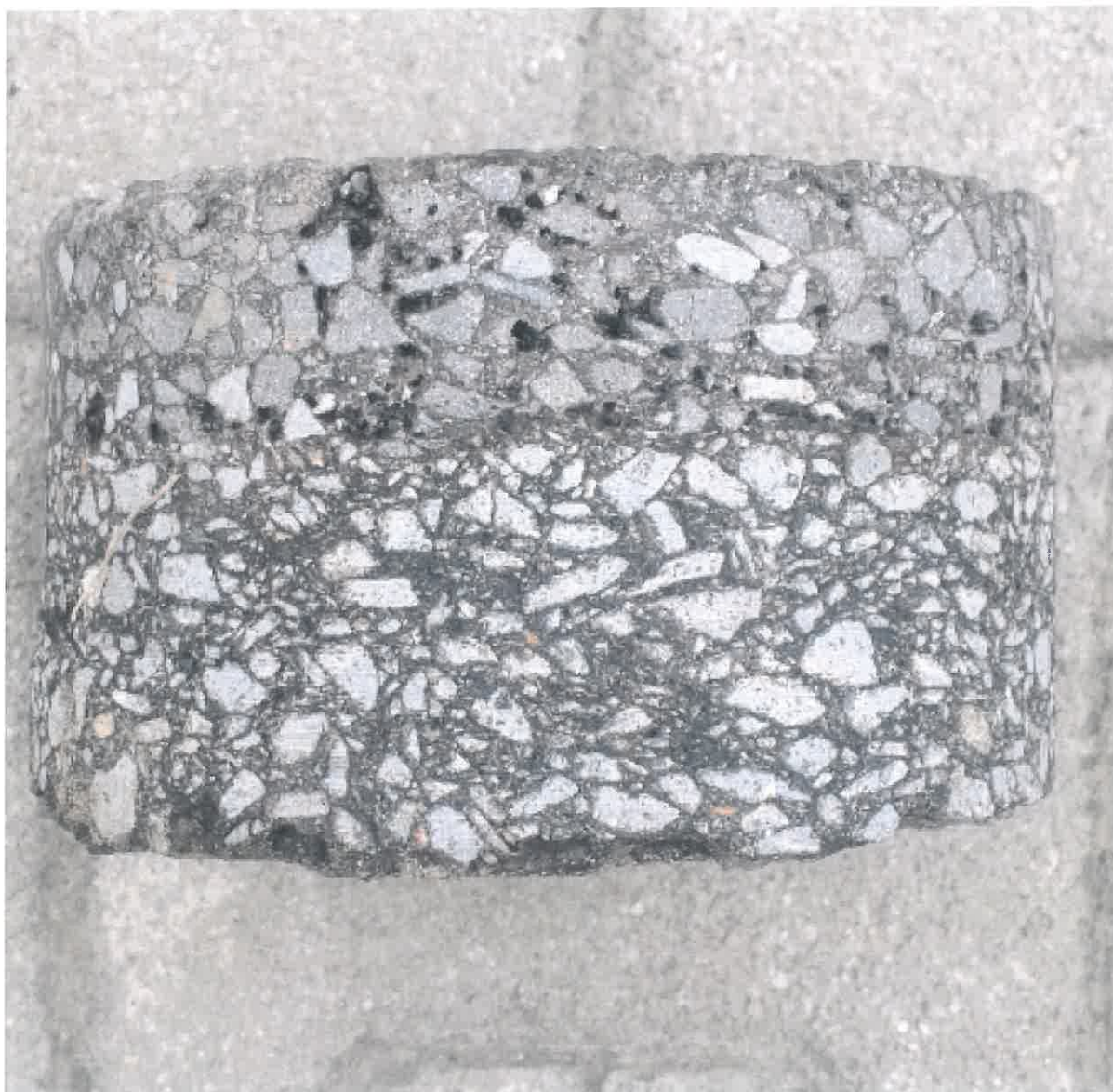
6. kép: Fúrt minta Nyíregyháza, Templom utca 1+150 km. sz. jobb oldal sávközép
