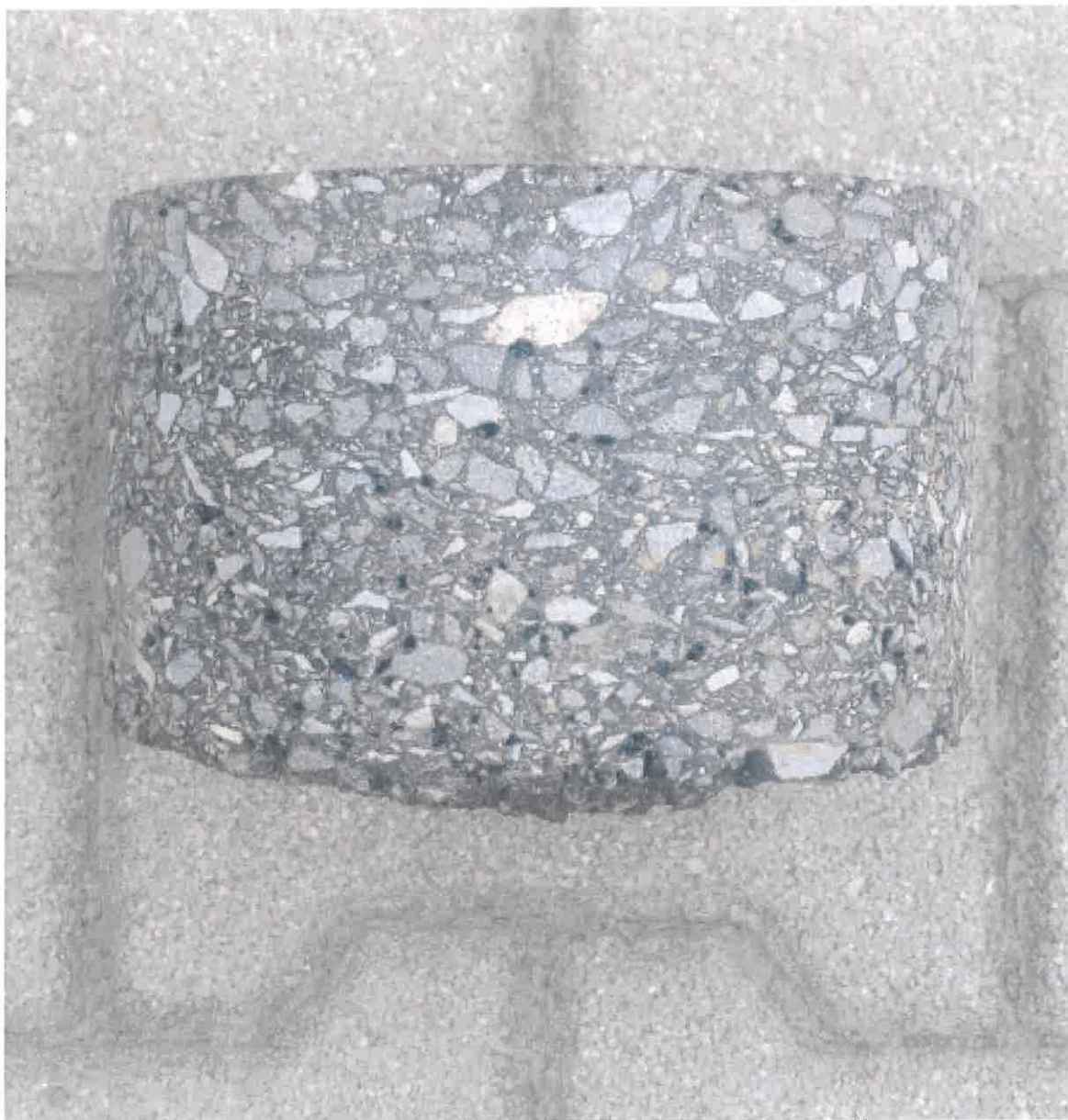
2. kép: Fúrt minta Nyíregyháza, Templom utca 0+475 km. sz. jobb oldal tengelytől 2,5 m
